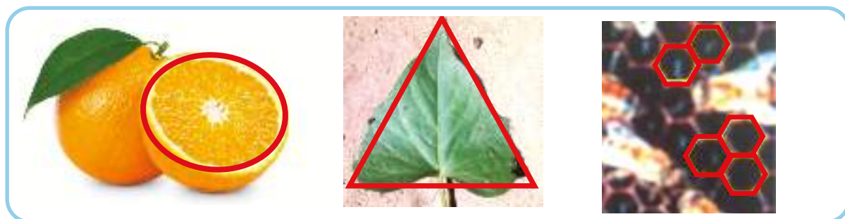
Figura 8 - Algumas formas geométricas na Natureza [circular, triangular e hexagonal].
