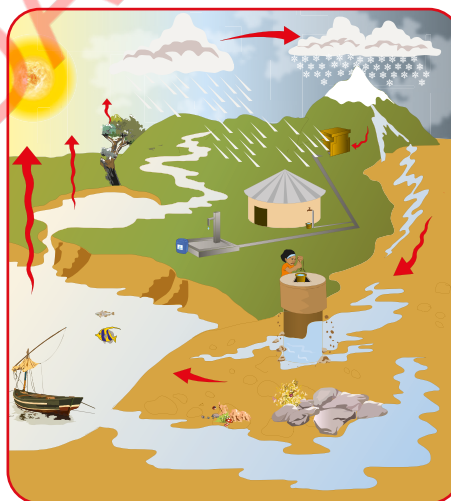
Figura 17 - Ilustração do ciclo da água
