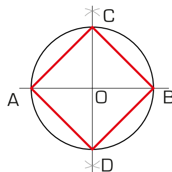
Figura 6 - Construção de um quadrado
